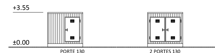
Façades pignons -
