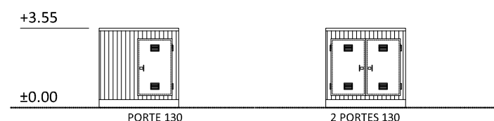
Façades pignons -
